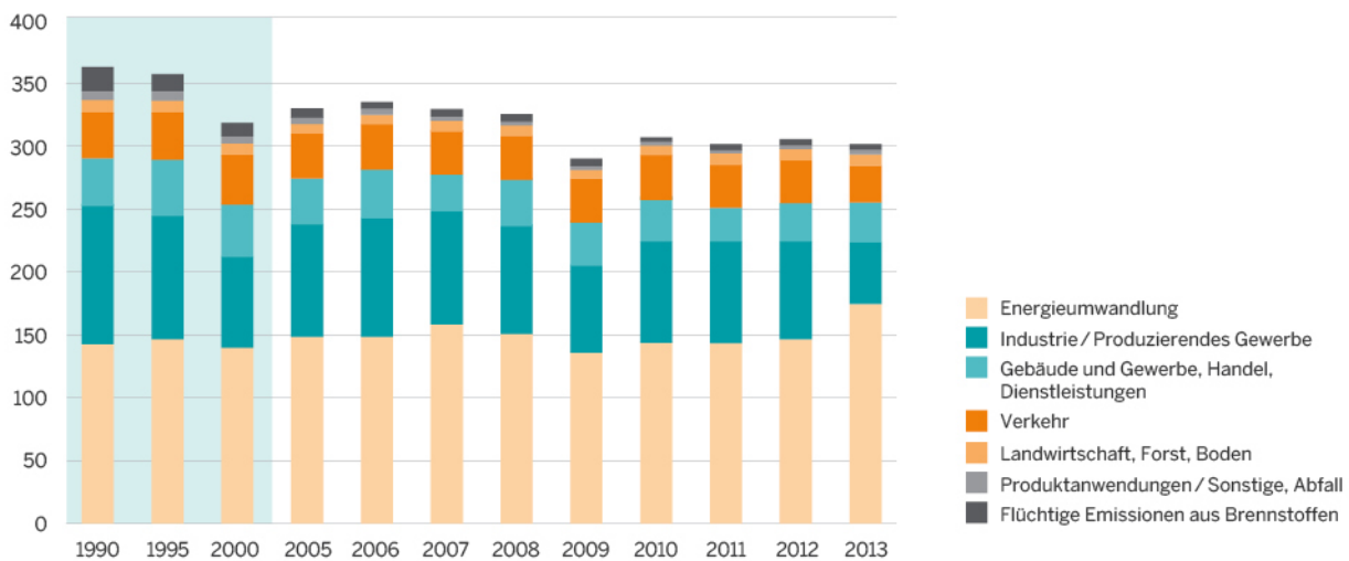
ENTWICKLUNG DER TREIBHAUSGASEMISSIONEN IN NRW VON 1990 BIS 2013. QUELLE: WUPPERTAL INSTITUT, LANUV, UMWELTBUNDESAMT (EIGENE DARSTELLUNG)
