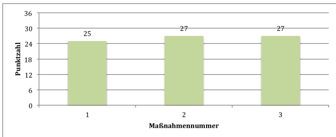
Abbildung 1: Bewertungsergebnisse
