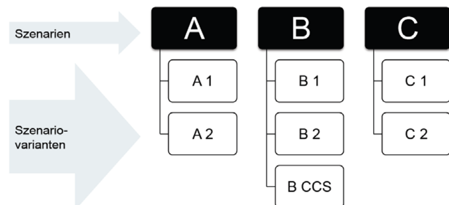
Abbildung 4: Übersicht zur Struktur der Szenarien des Klimaschutzplans
